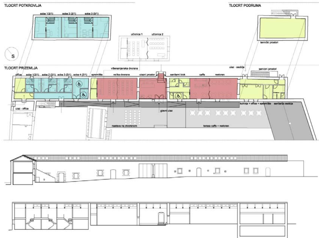
sl. 2. Međunarodni sveučilišni centar u Kuli Jankovića, Islam Grčki, Hrvatska studija idejnog rješenja
